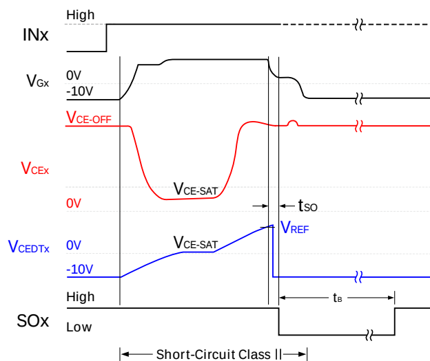
图 20. II 类短路监测信号波形
