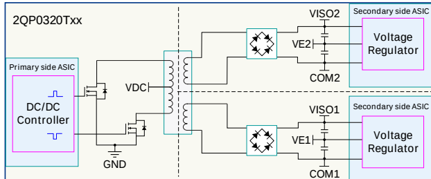
图 6. 供电电路
